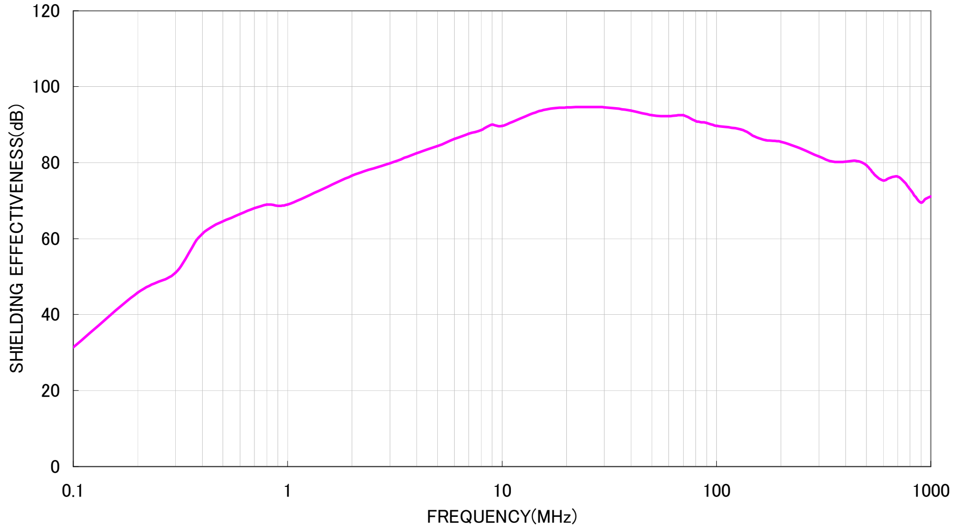
メタックス175C 電界シールドデータ(KEC法)
