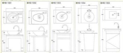
HD-1001 【手水鉢 W420×D360×H140】 セット価格 ¥340,200 (本体価格 ¥324,000)
