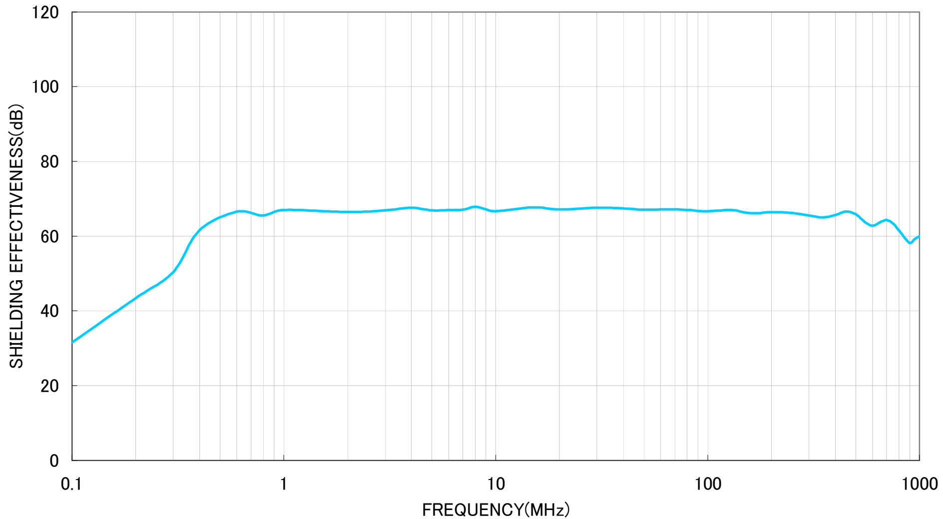
メタックス372N/C 電界シールドデータ(KEC法)
